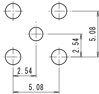
取付け穴寸法図
